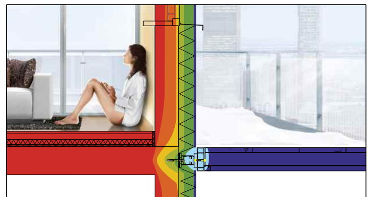
Abb. 2 Der neue Balkon Die Wärmedämmung der Wand ist aufrecht erhalten.
